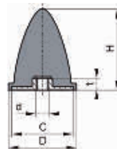
Typ EP: mit Innengewinde
