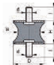
Typ A: beidseitig Gewindebolzen
