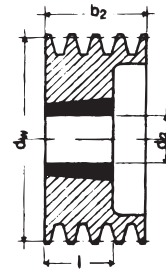
KEILRILLENSCHEIBEN
