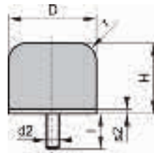
Typ 1G: ein Gewindebolzen
