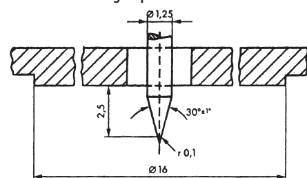
Eindringkörper nach Shore D
