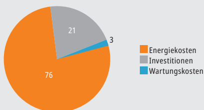
Kostenverteilung eines Druckluftsystems
