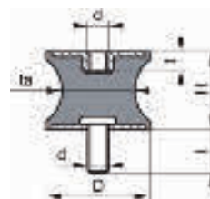
Typ B: Innengewinde/ Außengewinde
