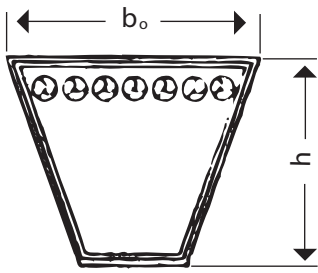
SCHMALKEILRIEMEN
