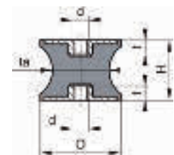
Typ C: Innengewinde
