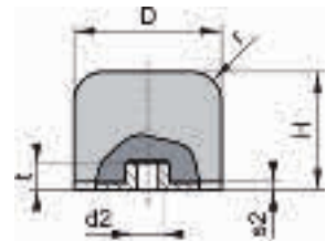
Typ IG: mit Innengewinde
