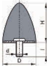
GUMMI-METALL-ANSCHLAG-PUFFER
