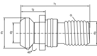
ISO 7388 II B (mit Bohrung)
