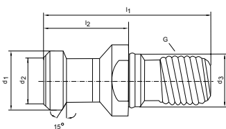
DIN 69872 A (mit Bohrung)
