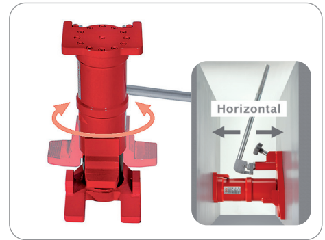
Hydr. Hebegerät Modell Unilifter U6 vertikaler/horizontaler Einsatz
